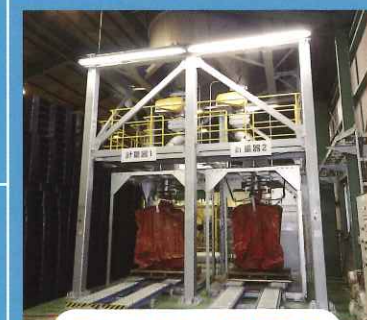
フレコンへの荷姿変更
